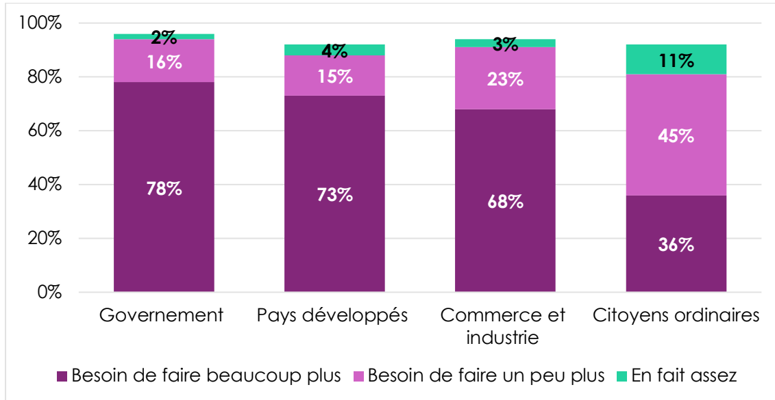
Figure 4 : Les acteurs font-ils assez pour limiter les changements climatiques ? | Zimbabwe | 2022
