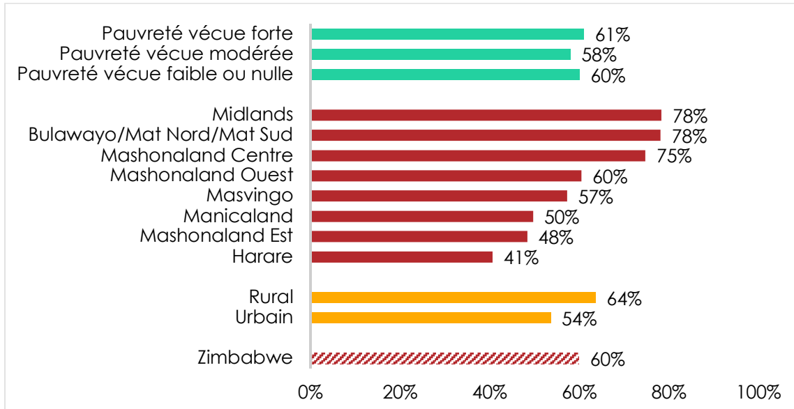
Figure 2 : Les sécheresses se sont aggravées | par groupe démographique | Zimbabwe | 2022
