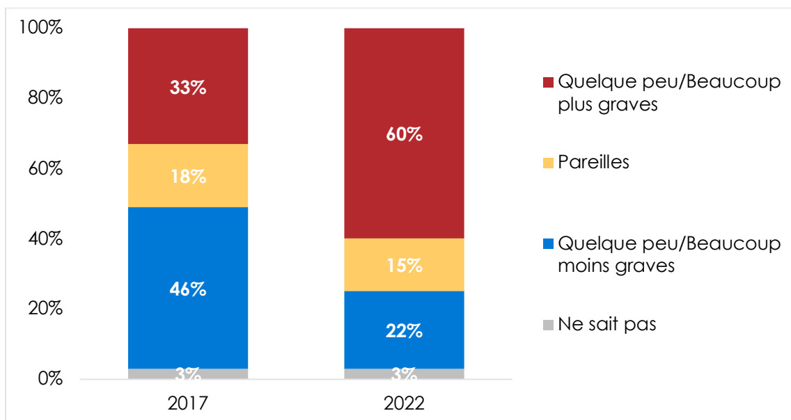
Figure 1 : Ampleur des sécheresses | Zimbabwe | 2017-2022
