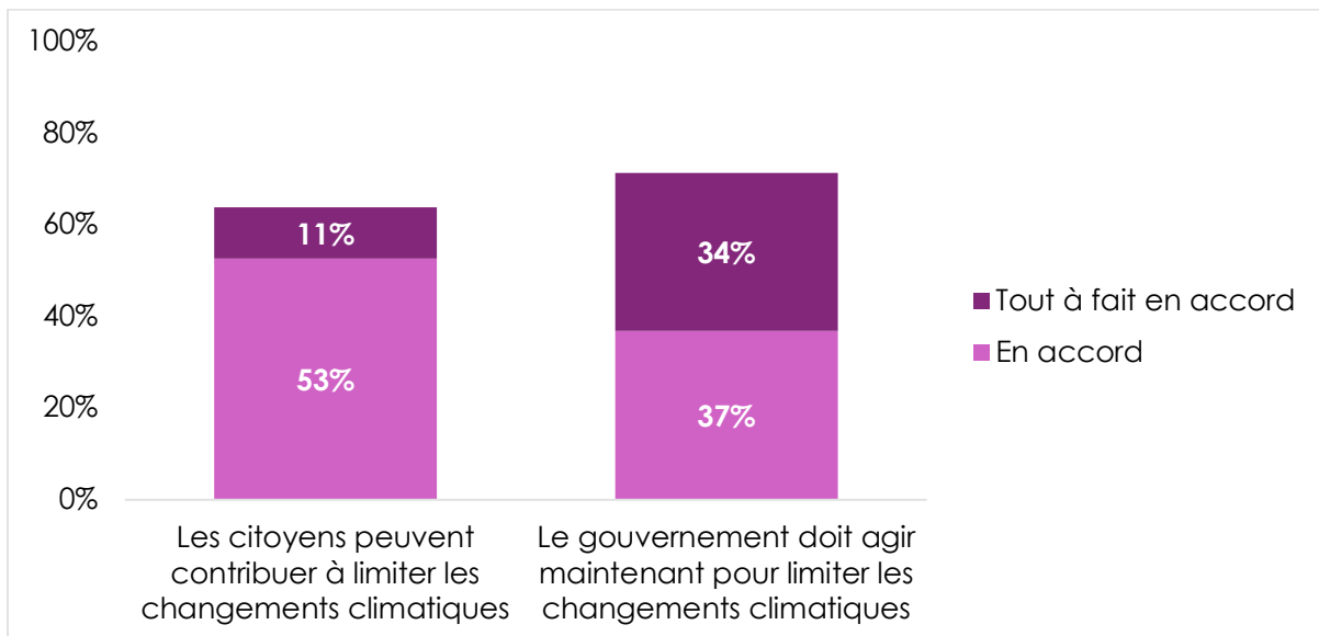
Figure 3 : Limiter les changements climatiques | Zimbabwe | 2022
