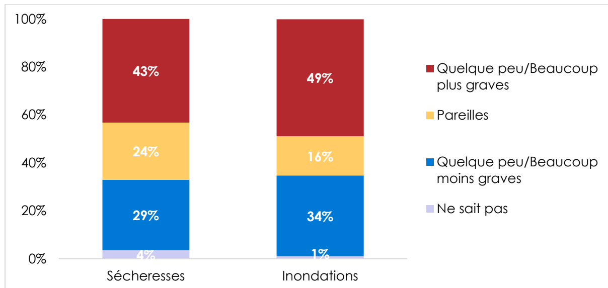
Figure 1 : Gravité des inondations et des sécheresses | Sénégal | 2022
