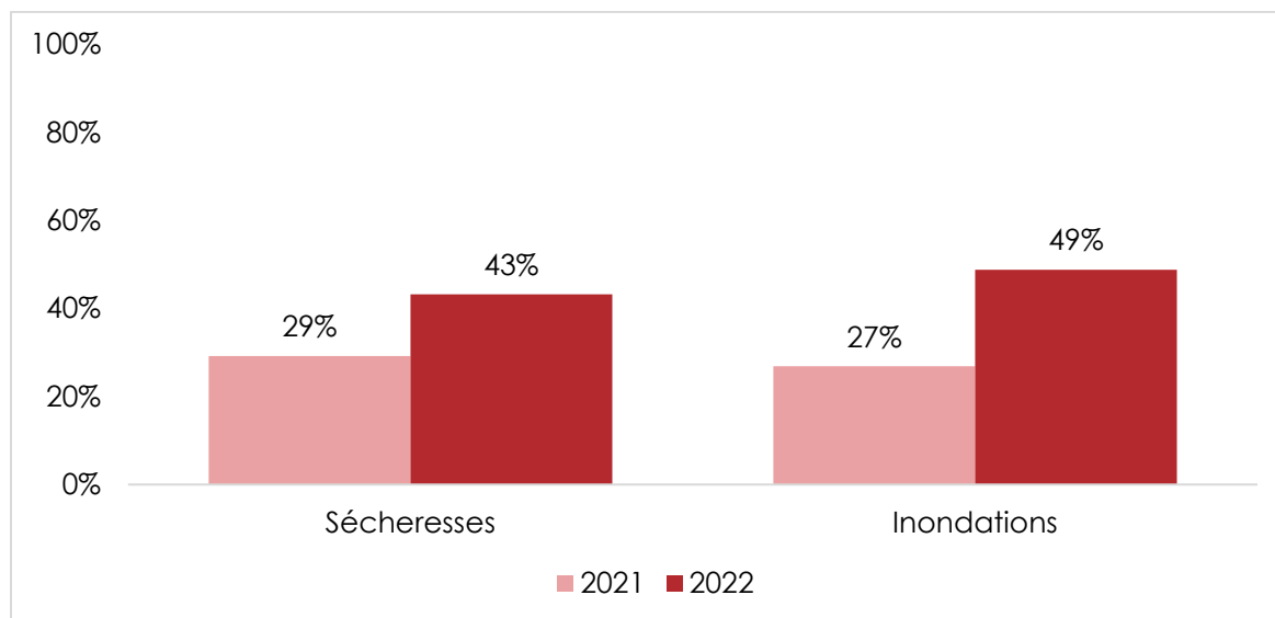
Figure 2 : Gravité croissante des inondations et des sécheresses | Sénégal | 2021-2022
